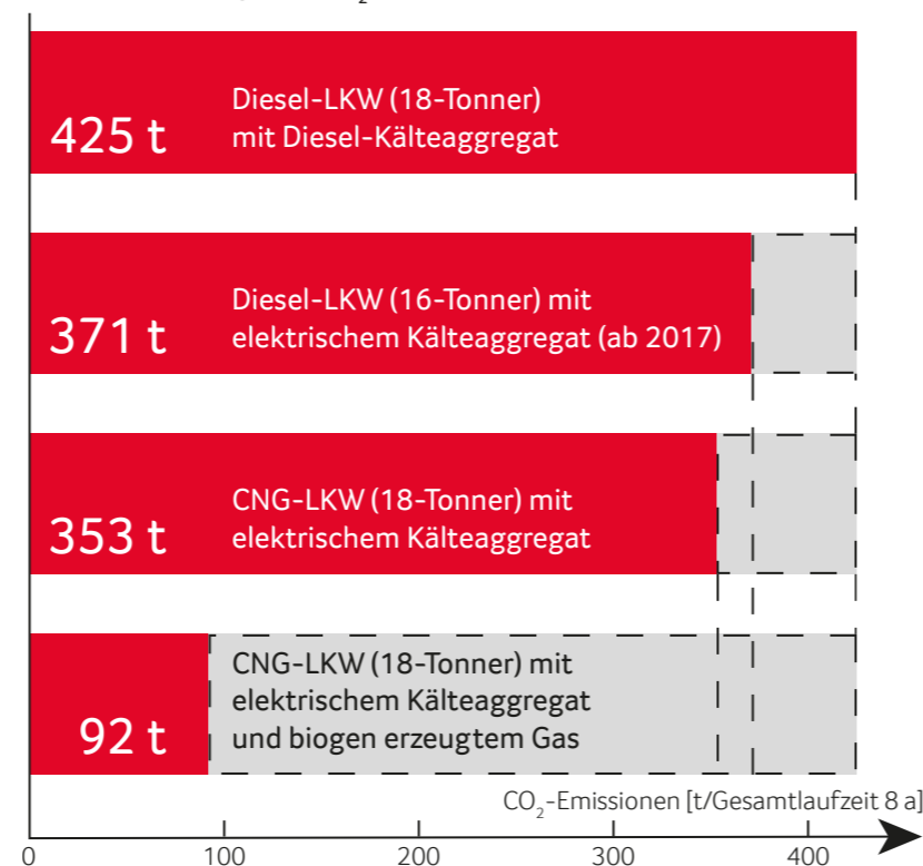
Vergleich CO 2 -Emissionen Diesel-LKW vs. CNG-LKW
